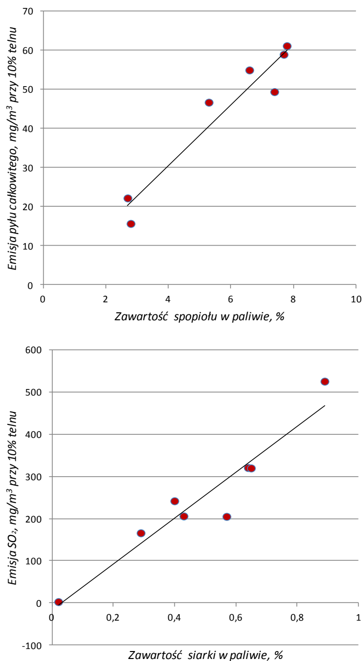
Rys. 27. Wpływa zawartości popiołu i siarki w węglu spalany w kotle z automatycznym załadunkiem paliwa na emisję pyłu oraz SO 2 (mg/m 3 przy 10% O 2 w spalinach) [K. Kubica; Właściwości węgla jako paliwa dla czystszej energii z kotłów węglowych małej mocy; Magazyn Instalatora; 01.2013]
