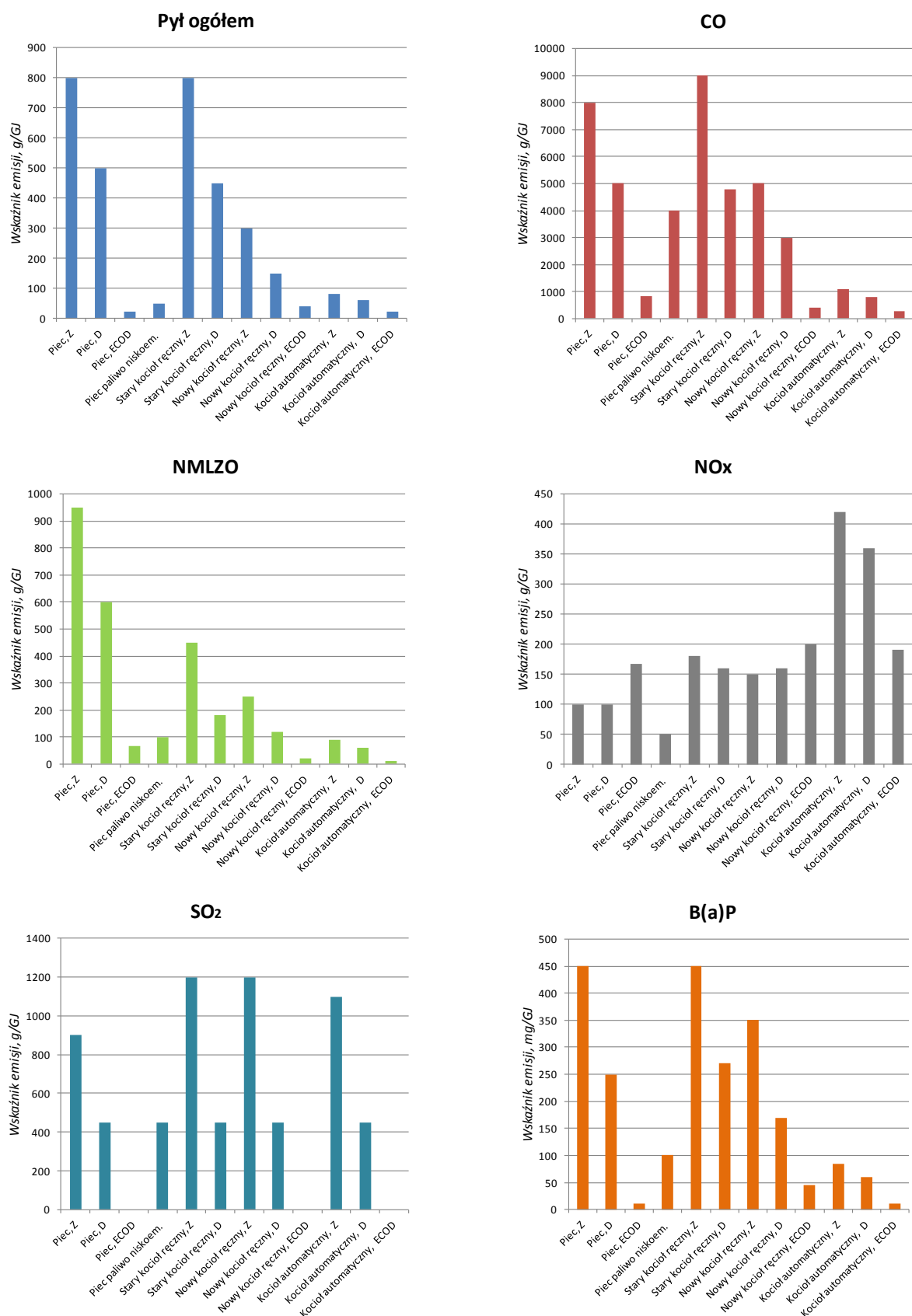
Rys. 17. Emisja zanieczyszczeń ze spalania węgla w różnych urządzeniach grzewczych Z – stara technika, D- nowa technika, ECOD – wymogi dyrektywy ErP
