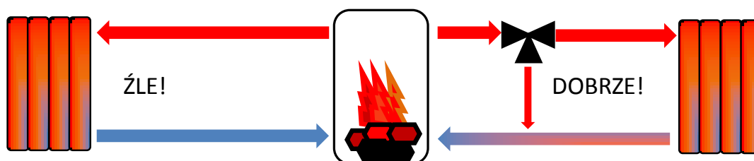
Rys. 36. Zastosowanie zaworu mieszającego
